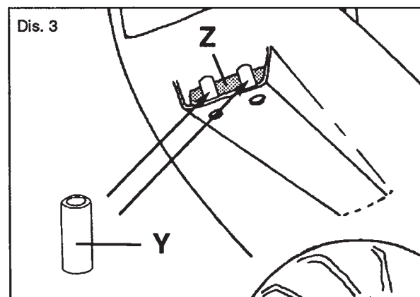
Dis. 3 - Inserire i distanziatori Y nel vano con la gommapiuma Z.
