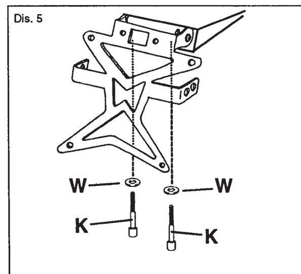
Dis. 5 - Inserire da sotto il codino le viti K con le rondelle W e bloccare il tutto.
