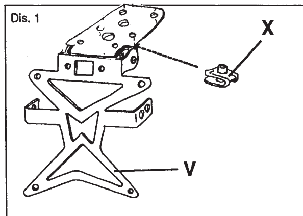
Dis. 1 - Montare le fascette X sul portatarga V con i fori in corrispondenza dei fori superiori della piastra mobile del portatarga V.
