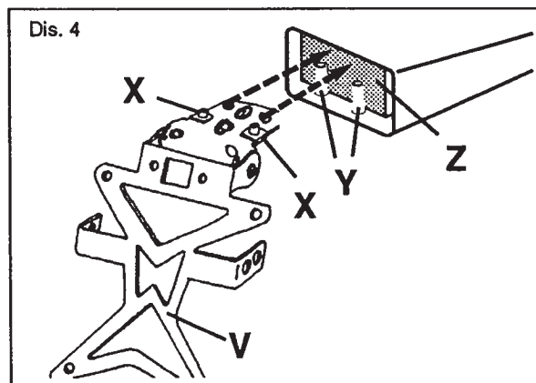
Dis. 4 - Inserire il portatarga V nel vano con la gommapiuma Z, con le fascette X posizionate sopra ai distanziatori Y.
